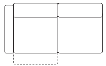
Laterale 3 posti da 192 Dx/Sx con 1 relax 3 seater Rh/Lh side element cm 192 with 1 relax L 192 P 101 H 81/99
