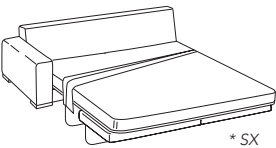
Laterale letto 3 posti da 190 Dx/Sx con rete elettrosaldata da 140 3 seater Rh/Lh side element cm 190 with 140 cm electro-welded net L 190 P 96/233 H 80
