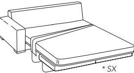
Laterale letto 2 posti maxi da 170 Dx/Sx con rete elettrosaldata da 120 2 maxi seater Rh/Lh side element cm 170 with 120 cm electro-welded net L 170 P 96/233 H 80
