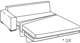
Laterale letto 2 posti maxi da 192 Dx/Sx con rete elettrosaldata da 140 2 maxi seater Rh/Lh side element 192 with 140 cm electro-welded net L 192 P 95/233 H 86
