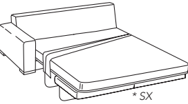
Laterale letto 2 posti maxi da 188 Dx/Sx con rete elettrosaldata da 140 2 maxi seater Rh/Lh side element cm 188 with 140 cm electro-welded net L 188 P 95/233 H 85
