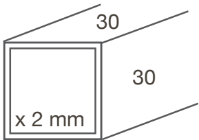
SEZIONE STRUTTURA BASE BASE STRUCTURE SECTION
