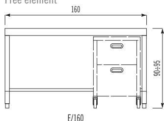
Elemento libero Free element
