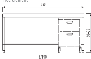
Elemento libero Free element
