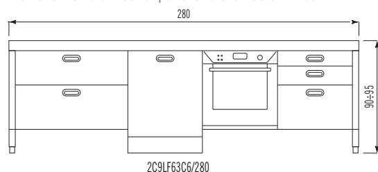
Elemento con pannello per lavastoviglie e forno da 60 cm Element with dishwasher panel and oven 60 cm wide
