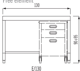
Elemento libero Free element
