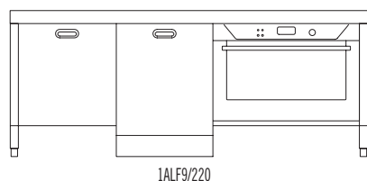
Elemento con pannello per lavastoviglie e forno da 90 cm Element with dishwasher panel and oven 90 cm wide
