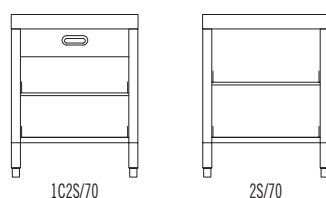
Elementi aperti con ripiani scorrevoli Open elements with sliding shelves
