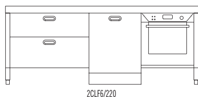
Elemento con pannello per lavastoviglie e forno da 60 cm Element with dishwasher panel and oven 60 cm wide
